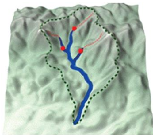
चित्र 4.5 : अपवाह प्रणाली
