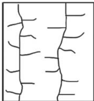
चित्र 4.8 : आयताकार प्रतिरूप
