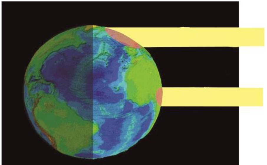
चित्र 3.1: अक्षांश के अनुसार किरणों का फैलाव
