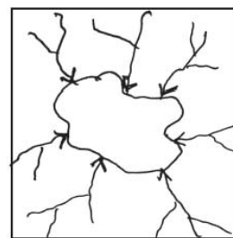
चित्र 4.9 : केन्द्रोन्मुखी प्रवाह प्रतिरूप
